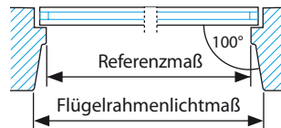
Skizze 2 – z.B. Roto-fenster mit Glasleiste schräg/gerade
