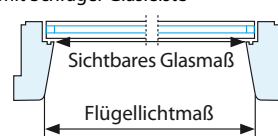
Skizze 2 – z.B. Roto-Fenster mit Glasleiste schräg/gerade
