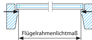
Skizze 2 – z.B. Roto-fenster mit Glasleiste schräg/gerade
