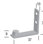
Spannwinkel für Seitenführung SF inkl. Spannmuffe (Lieferumfang bei Option SF)
